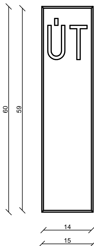
Szemből nézet
