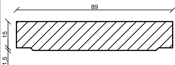
Keresztmetszet
