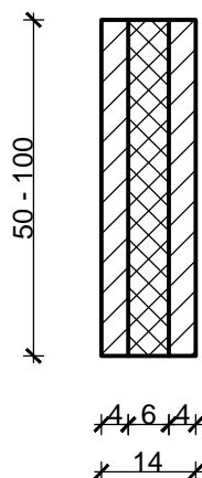
Keresztmetszet
