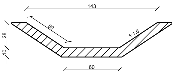
Keresztmetszet
