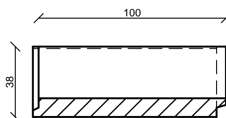
Hosszmetszet
