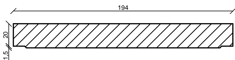
Keresztmetszet
