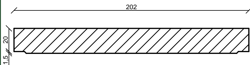
Keresztmetszet
