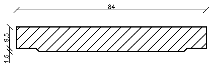
Keresztmetszet
