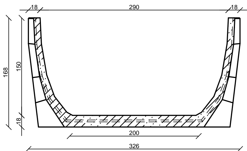
Keresztmetszet
