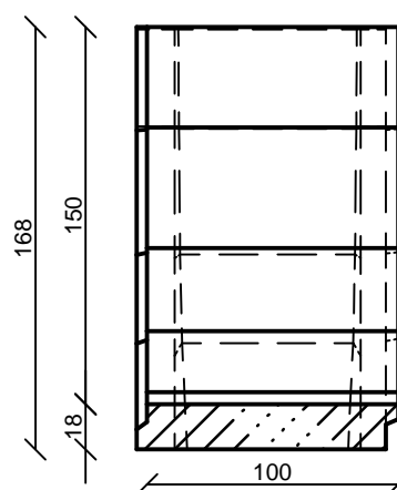
Hosszmetszet
