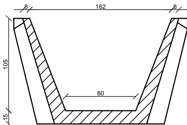
Keresztmetszet
