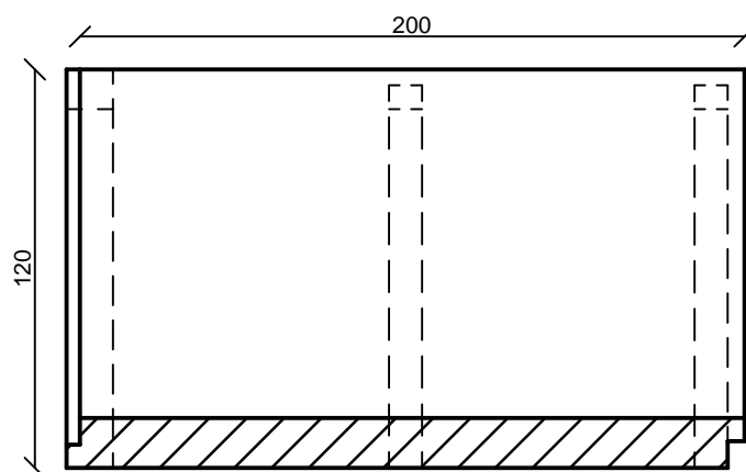
Hosszmetszet
