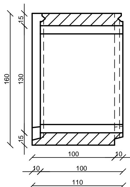
Hosszmetszet
