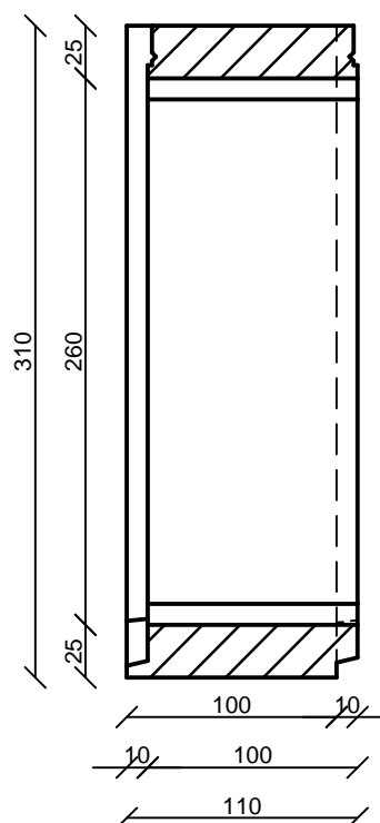
Hosszmetszet
