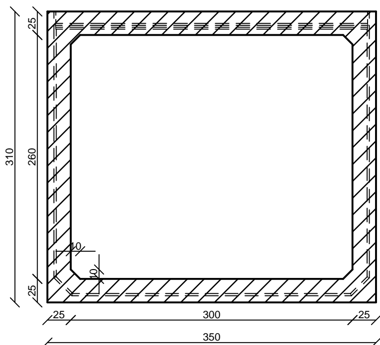
Keresztmetszet
