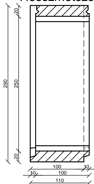
Hosszmetszet
