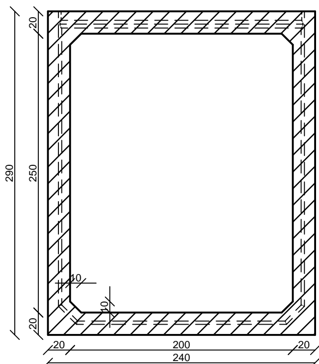
Keresztmetszet
