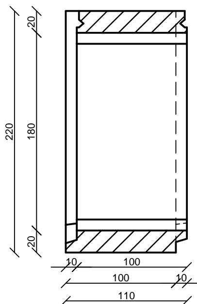
Hosszmetszet
