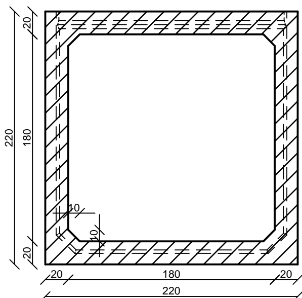
Keresztmetszet
