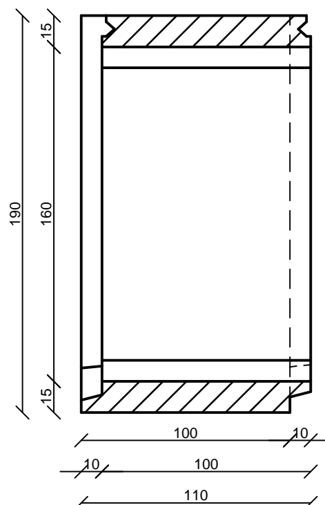
Hosszmetszet
