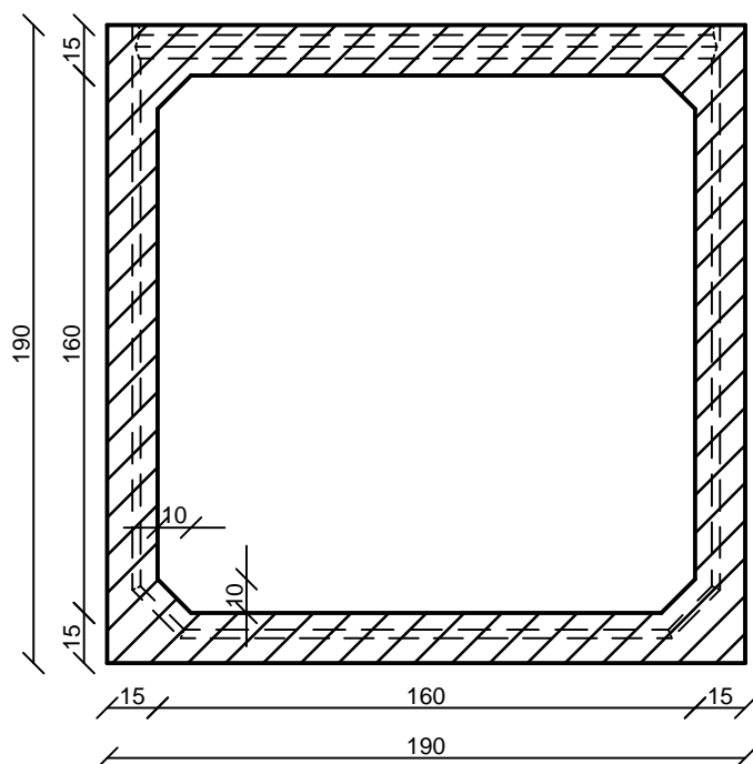
Keresztmetszet
