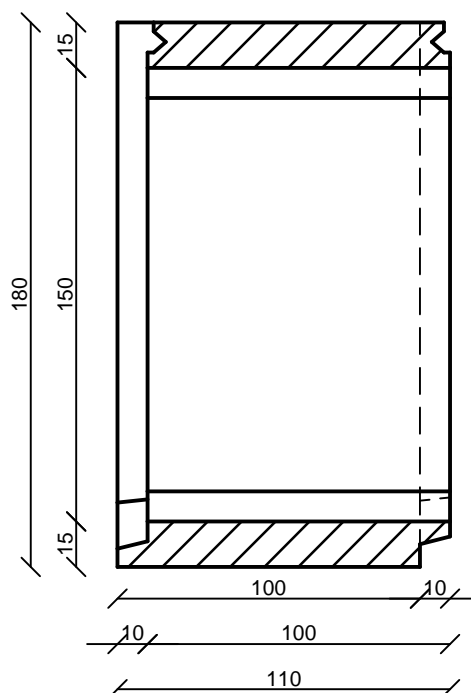
Hosszmetszet
