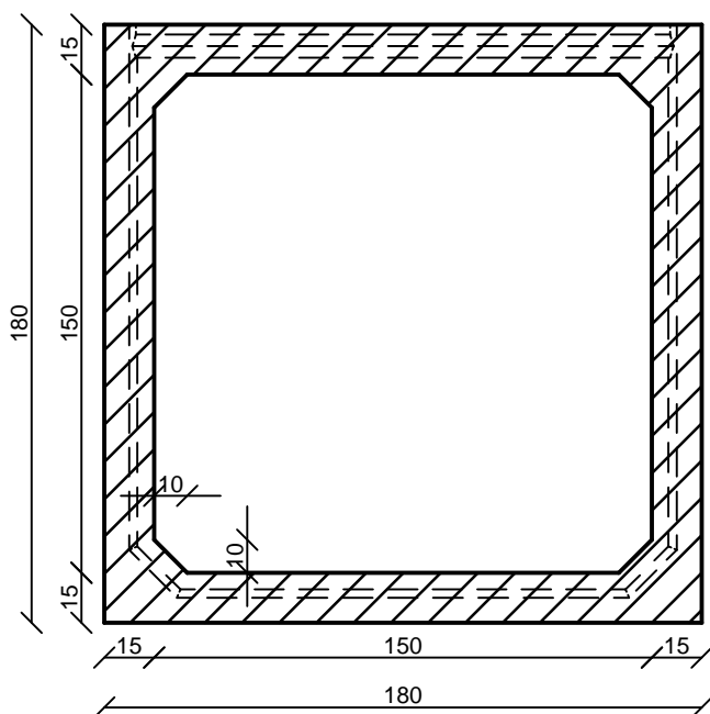
Keresztmetszet
