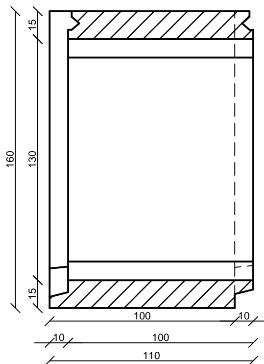
Hosszmetszet
