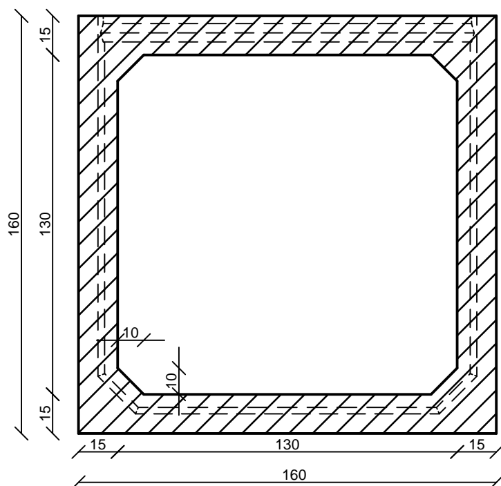
Keresztmetszet
