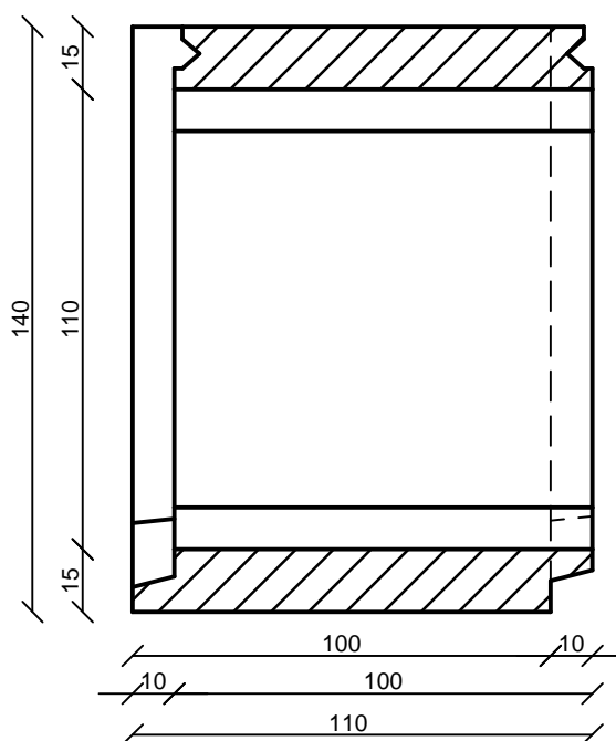
Hosszmetszet
