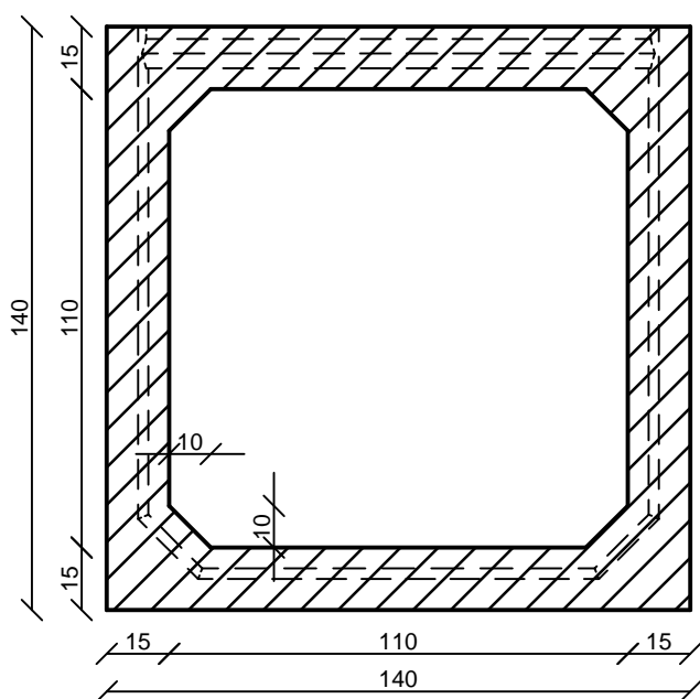
Keresztmetszet
